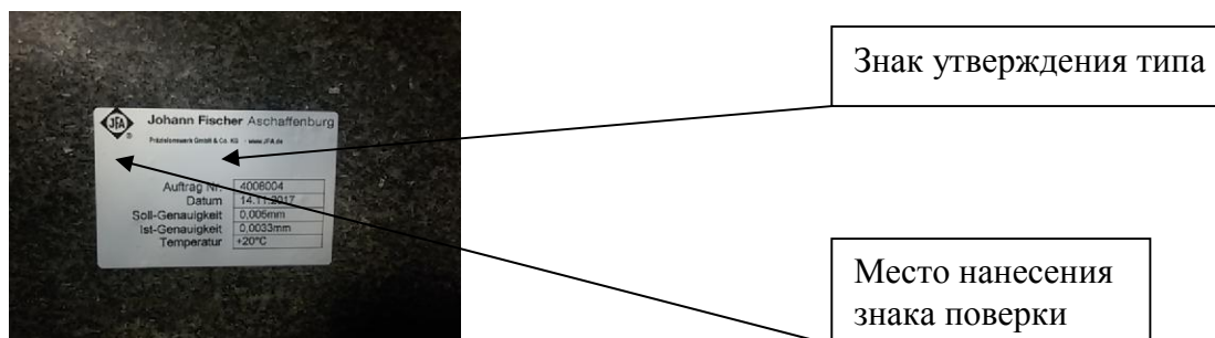
Рисунок 2 – Места нанесения знака поверки и знака утверждения типа
