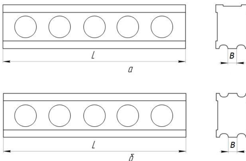
Рисунок 8 - Общий вид брусков модели 8 и обозначение их основных размеров а – с одной рабочей поверхностью; б – с двумя рабочими поверхностями
