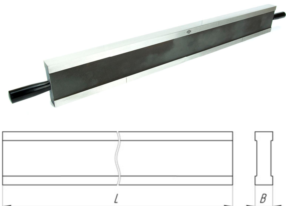
Рисунок 3 - Общий вид брусков модели 3 и обозначение их основных размеров
