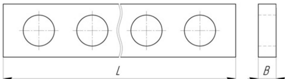
Рисунок 2 - Общий вид брусков модели 2 и обозначение их основных размеров
