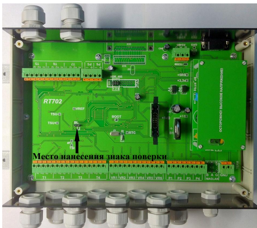
Рисунок 5 – Схема пломбировки от несанкционированного доступа, обозначение места нанесения знака поверки на переключатель, расположенную на плате вычислителя без встроенного регистратора расхода
