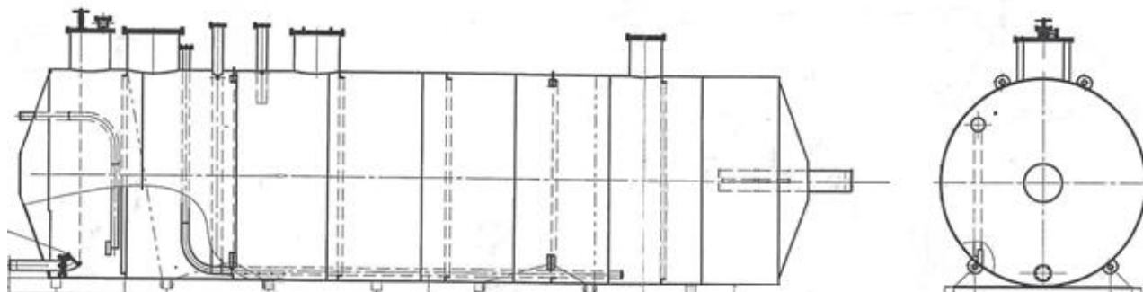
Рисунок 1 - Эскиз РГС-100
