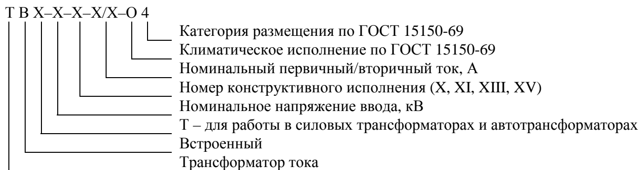
Рисунок 3 – Структура условного обозначения трансформаторов тока серий ТВТ и ТВ
