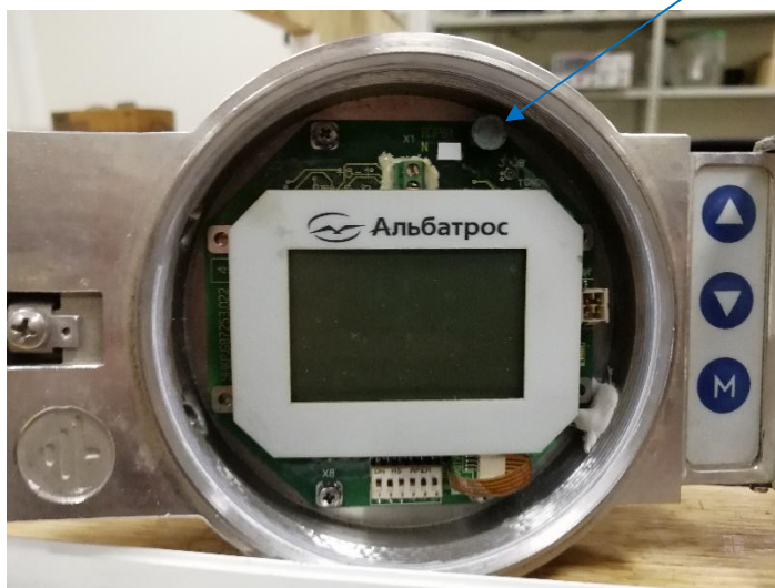
Рисунок 2 – Схема пломбировки
