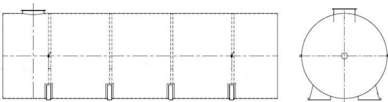
Рисунок 1 – Эскиз резервуара
