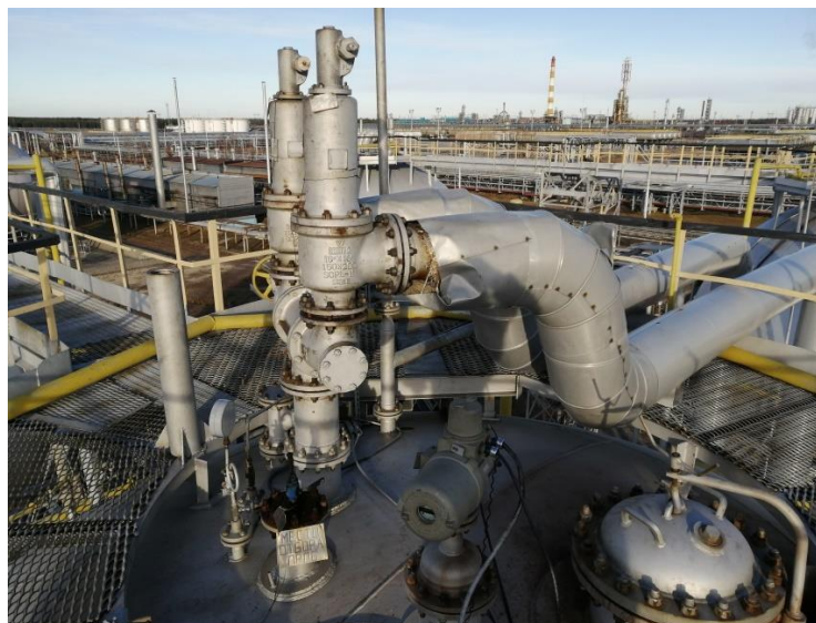
Рисунок 9 – Общий вид резервуаров РШС-600
