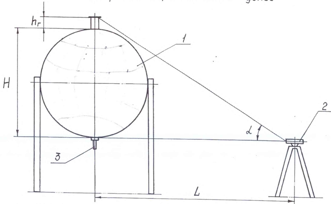
1- шаровой резервуар; 2- теодолит; 3- отвес с магнитным держателем Черт. 3
