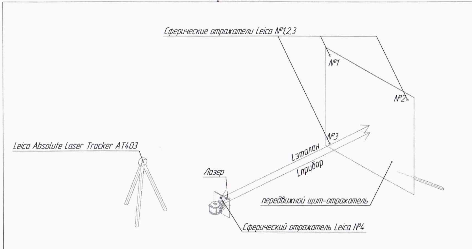
Рисунок А.1 – Схема подключения эталонной установки и поверяемого уровнемера
