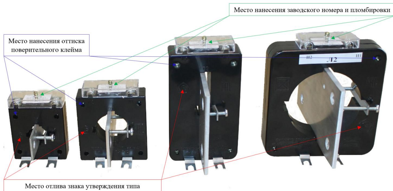
Рисунок 1 – Общий вид трансформаторов тока ТШП-0,66 У3 с указанием мест пломбировки, знака утверждения типа, нанесения заводского номера и отиска поверительного клейма
