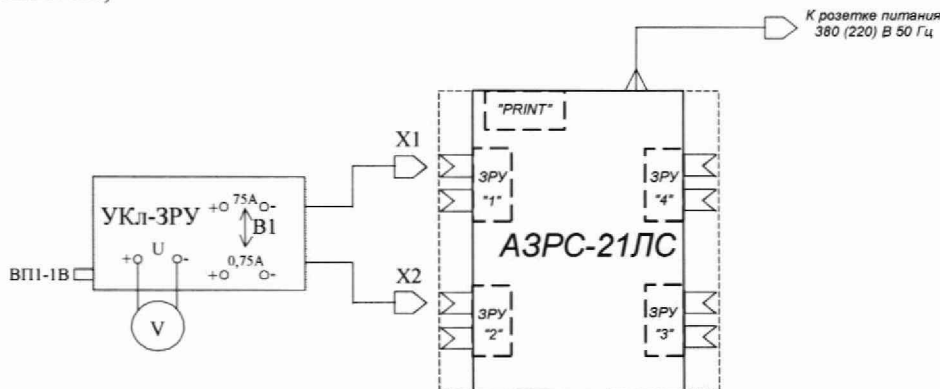
УКл-ЗРУ – устройство калибровочное, V – мультиметр В7-81, ВП1-1В – вставка плавкая (предохранитель)
