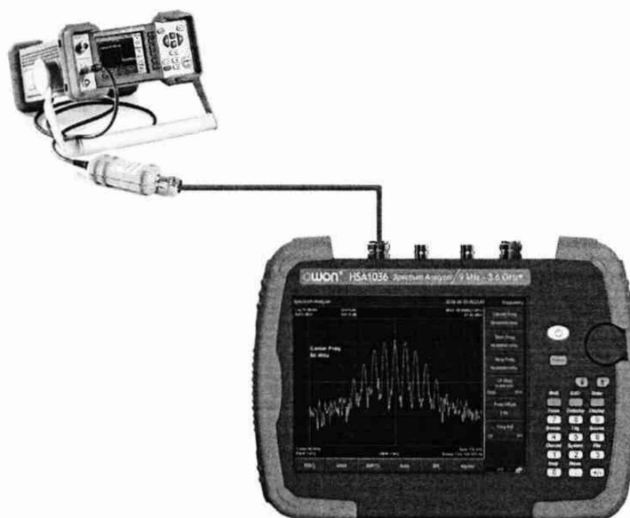
Рисунок 5 – Схема соединения приборов для определения абсолютной погрешности установки опорного уровня следящего генератора
