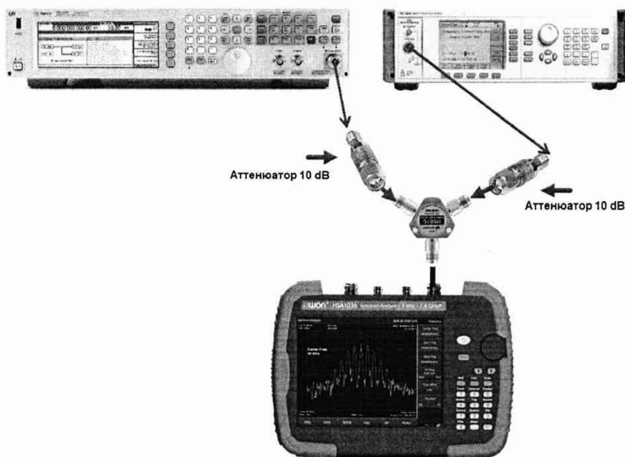
Рисунок 4 - Схема соединения приборов для определения уровня интермодуляционных искажений 3-го порядка
