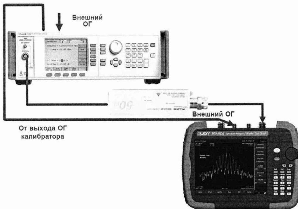
Рисунок 3 – Схема соединения приборов для определения относительной погрешности установки полос пропускания
